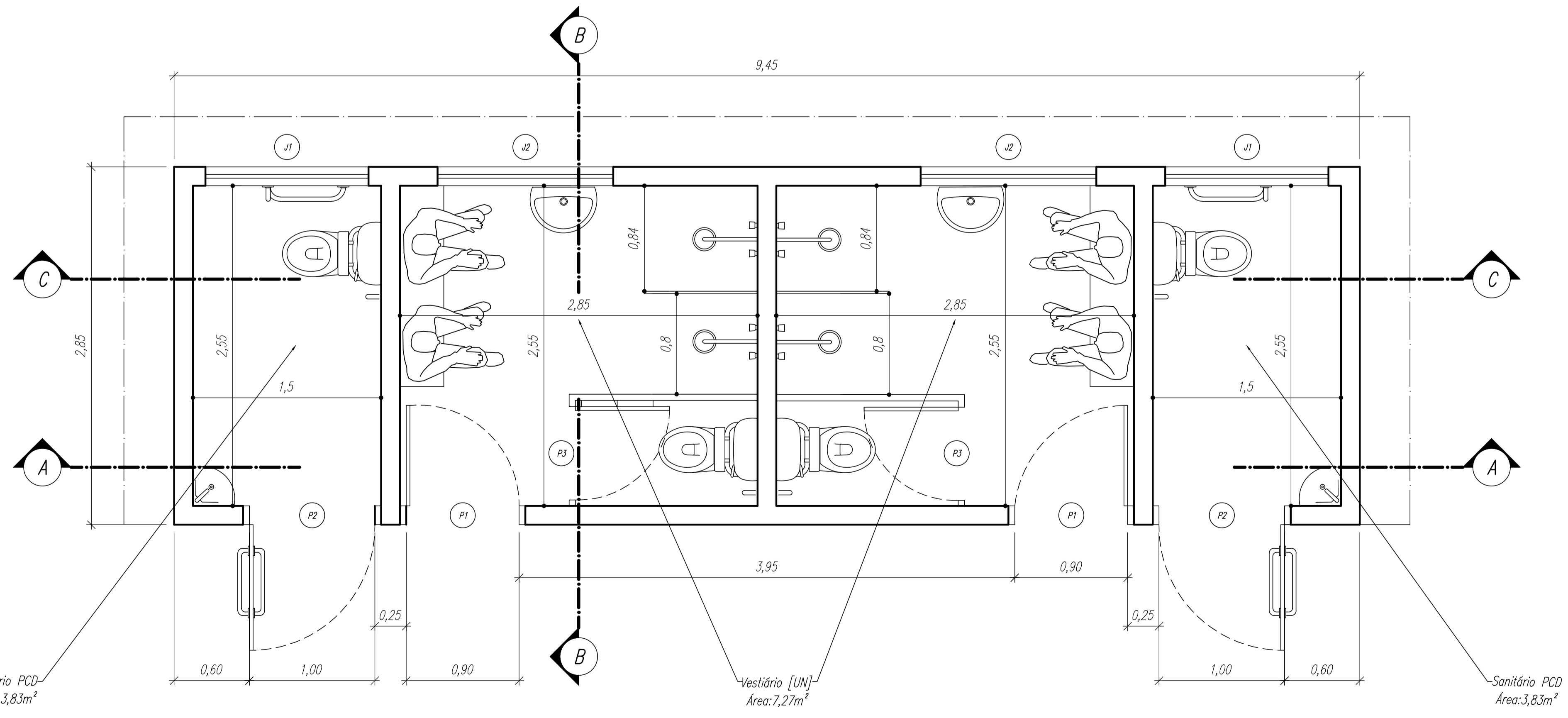
2 PLANTA DO VESTIÁRIO ESCALA - 1:25
