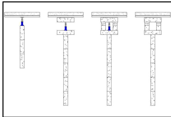
Figura 2 – Ilustração do procedimento de cravação da Estaca Mega.
