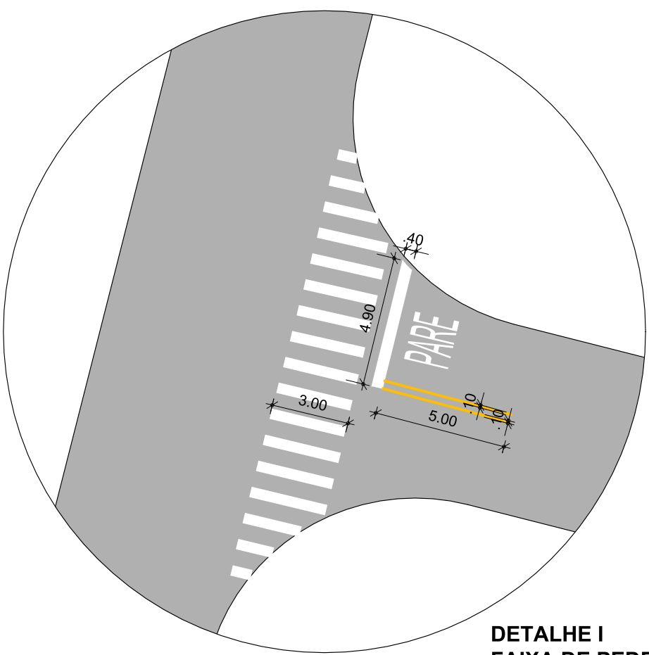
DETALHE I FAIXA DE PEDESTRE LINHA RETENÇÃO FAIXA DUPLA S/ ESCALA
