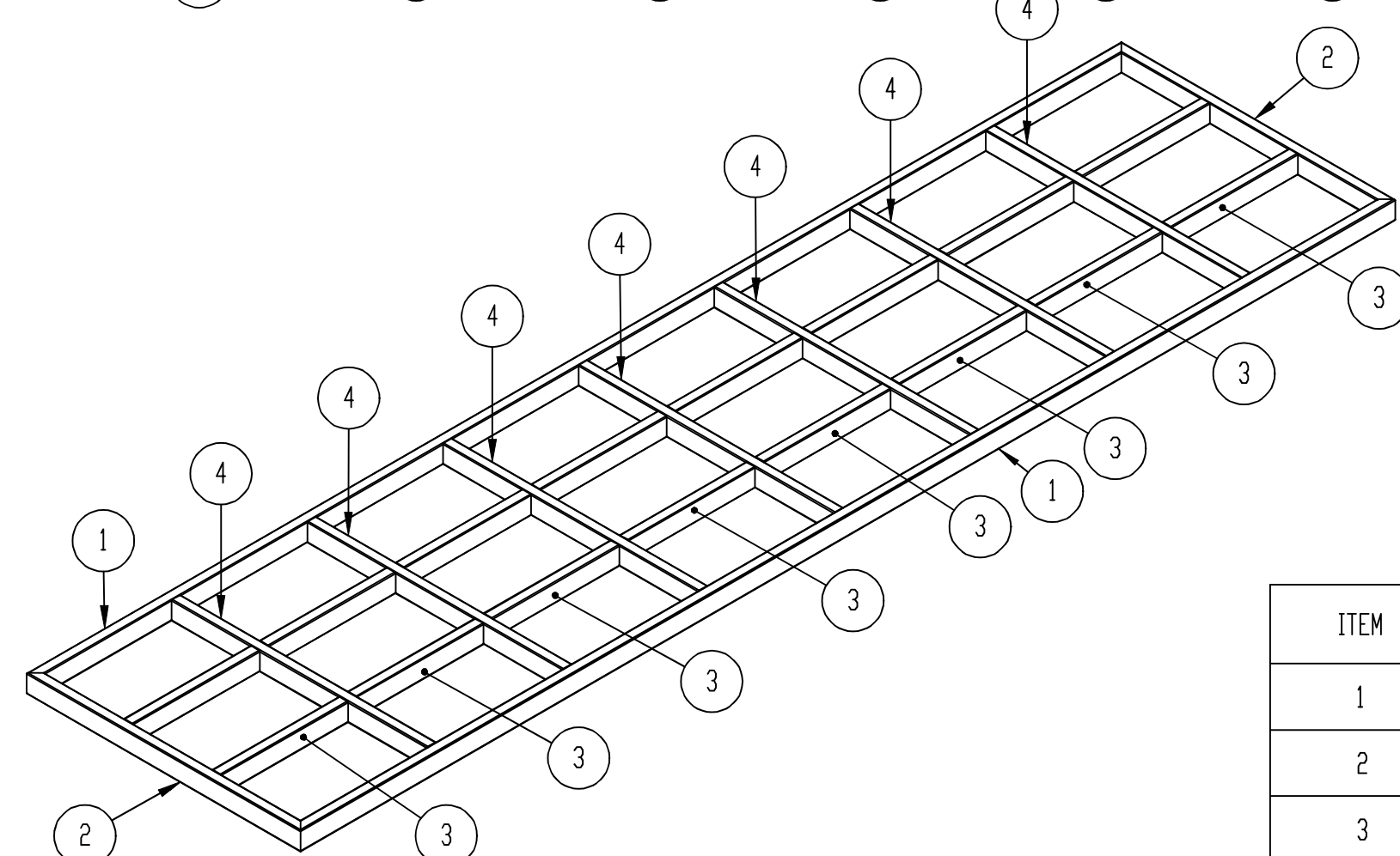
DETALHE ESTRUTURA SOLDADA PASSARELA ESCALA 1 : 25
