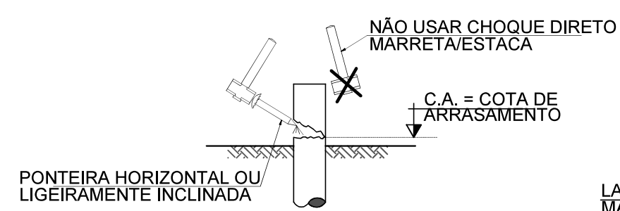
DETALHE P/ PREPARO DA CABEÇA DAS ESTACAS SEM ESC.
