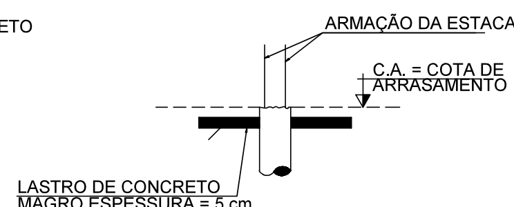
DETALHE P/ PREPARO DO BLOCO DE COROAMENTO SEM ESC.
