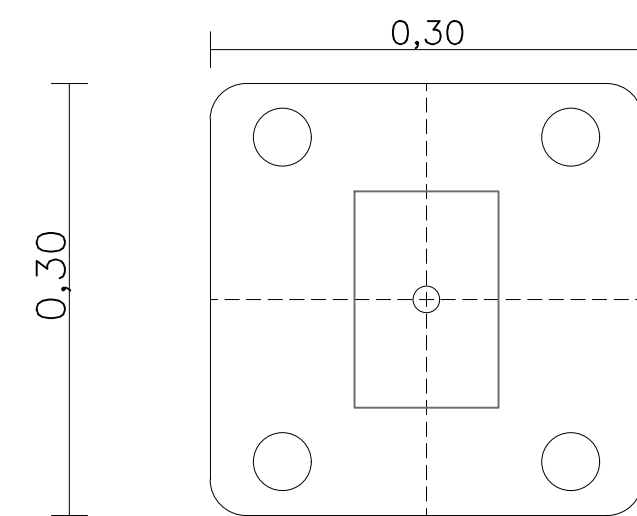
CHAPA PARA BASE DO PARABOLT ESC 1:50
