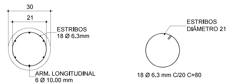
RESUMO DO AÇO - ESTACAS Ø30CM - UNITÁRIO
