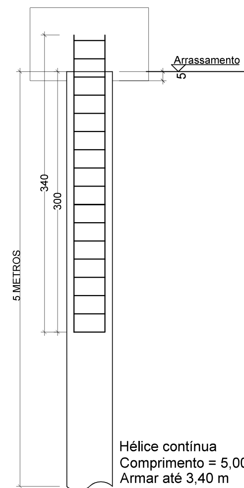
2 PERFIL - ESTACA COM D = 30CM SEM ESCALA
