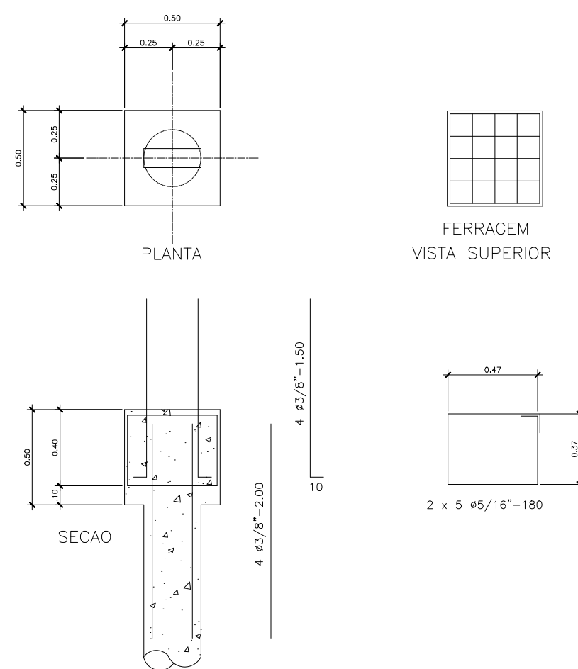
BLOCO - 01 ESTACA SEM ESCALA
