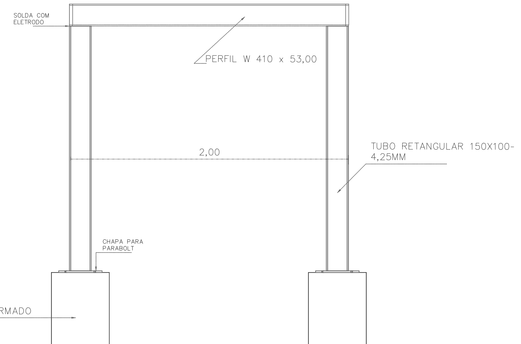
BLOCOS SOBRE 01 ESTACA SEM ESCALA
